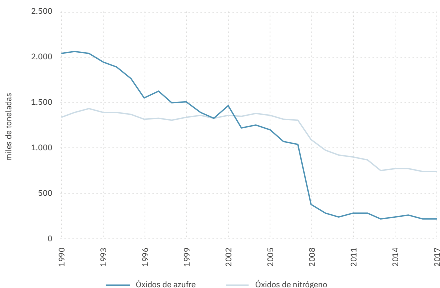
Fig. 12. Emisiones de contaminantes atmosféricos
